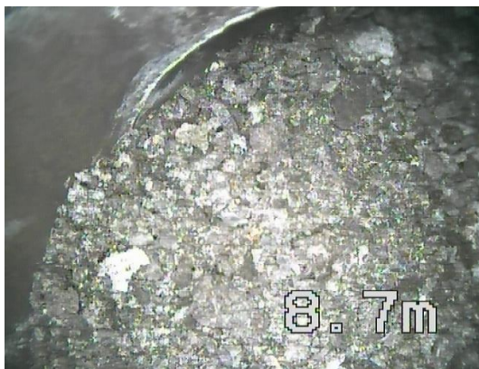
Rookgasbuis verstopt
